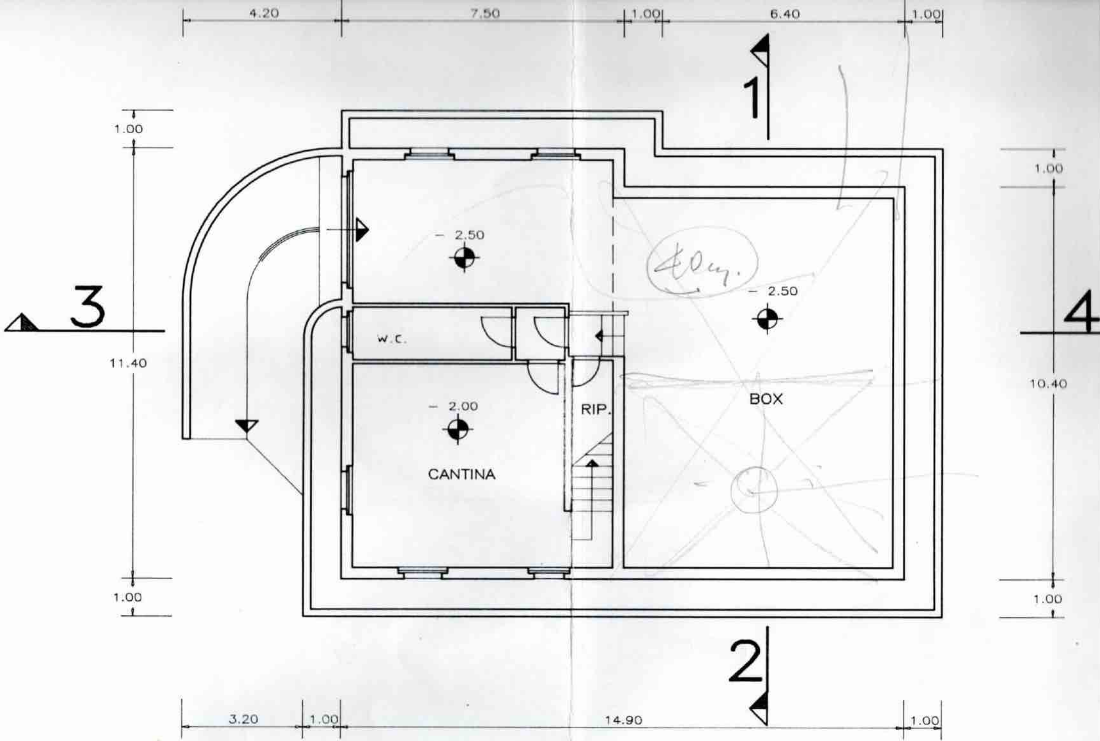
PIANTA PIANO SEMINTERRATO
