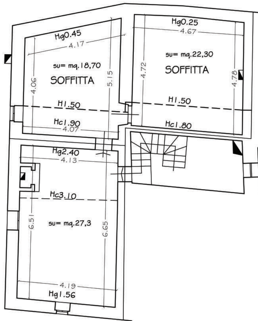
PIANTA PIANO SECONDO/SOTTOTETTO
