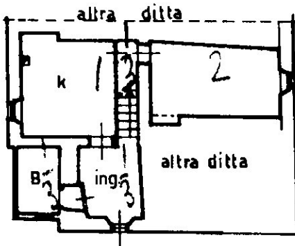
PIANTA PIANO TERRA H=2,28
