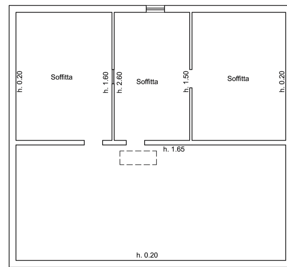
Pianta Soffitte
